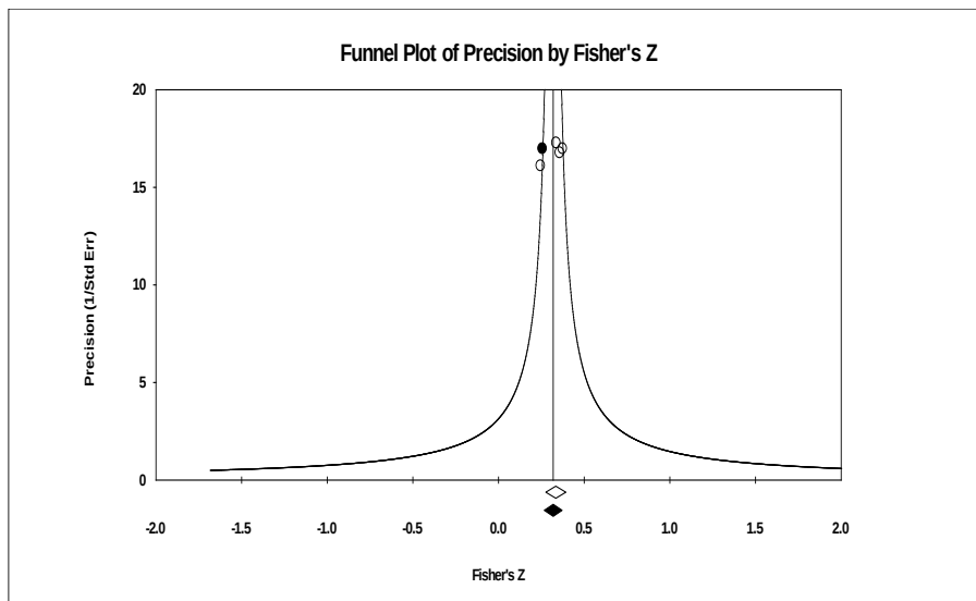
نمودار ۳: نمودار فانل (قیفی) دقت استاندارد براساس Z فیشر
