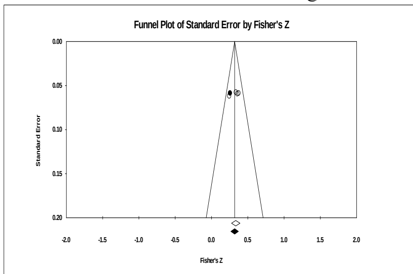
نمودار ۲: نمودار فانل (قیفی) تحقیقات عوامل مؤثر در فرسودگی شغلی (خطای استاندارد براساس Z فیشر)
