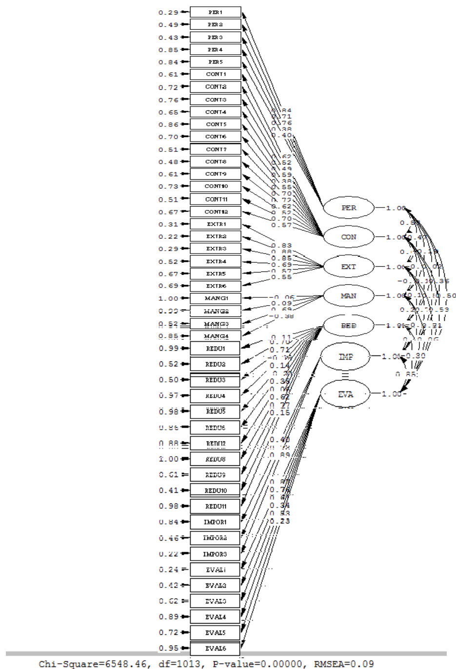
شکل ۱: نتایج تحلیل عاملی در حالت تخمین استاندارد
