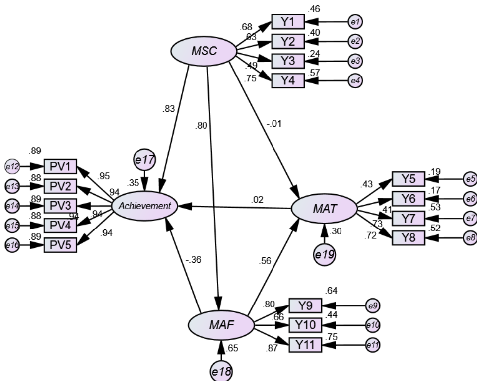
شکل ۳: مدل معادلات ساختاری میان خودپنداره ریاضی، نگرش، علاقه به ریاضی و متوسط پیشرفت ریاضی در تیمز
