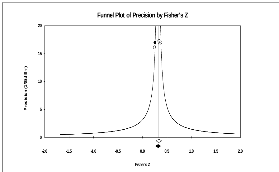
نمودار ۳: نمودار فائل (قیفی) دقت استاندارد براساس Z فیشر
